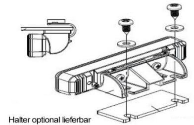
Heckmontage
