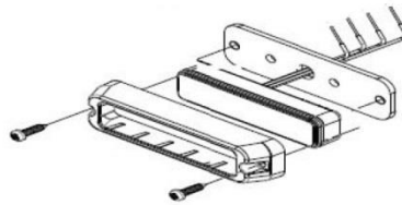
Frontmontage
